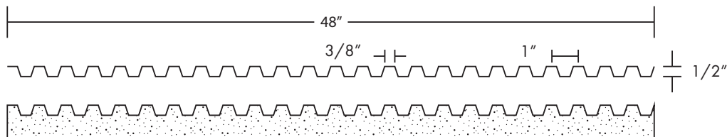
Section A-A
