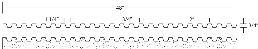
Section A-A
